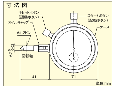
HL 低速・高速切替式 目量5/0.5rpm 測定範囲0~10,000rpm 0~1,000rpm
