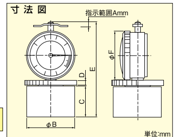
TM-106YS 目量0.01mm 測定範囲99~113mm
