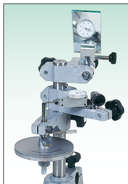
使用例 てこ式ダイヤルゲージの検査
