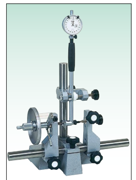
使用例 シリンダゲージの検査
